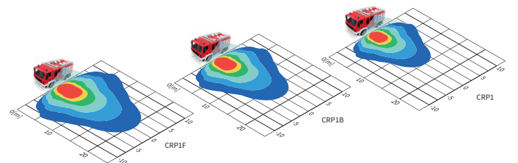
Beleuchtungsstärke von 1lx ermöglicht das Lesen in einer Zeitung Position des Scheinwerfers: h=2,5m
